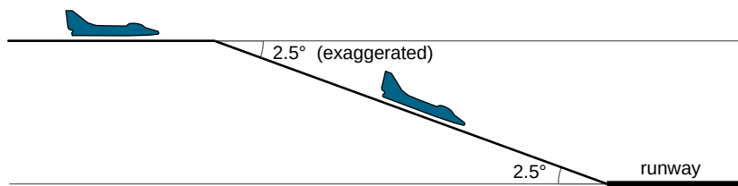
Abbildung 8.38: Glideslope
