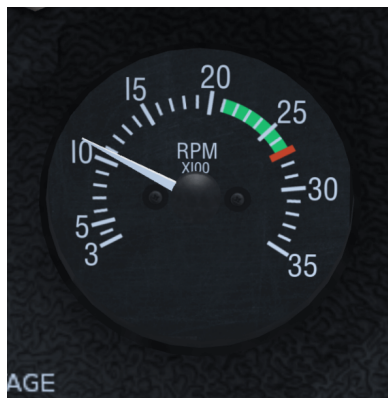
Abbildung 8.17: Tachometer
