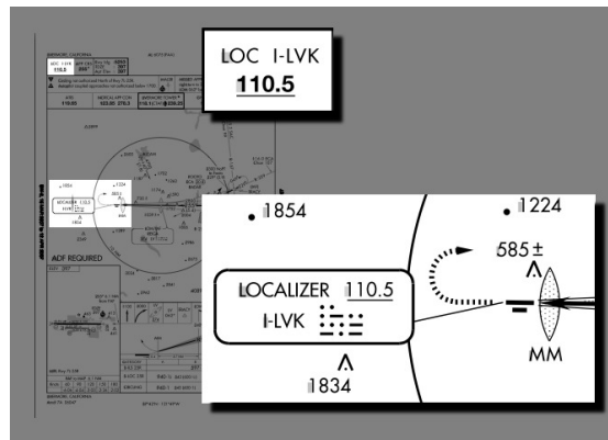
Abbildung 10.16: Livermore 25R localizer
